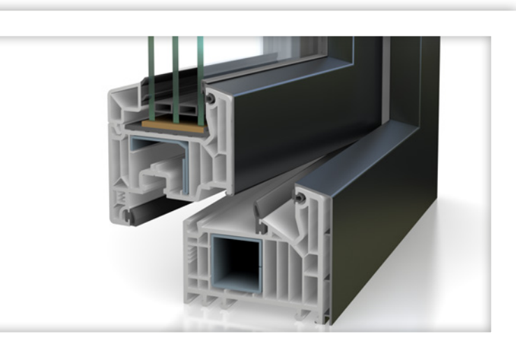
Perfekte Verbindung: Die individuell gestalteten Aluminium-Vorsatzblenden verdecken die Kunststoffprofile von außen vollständig.
